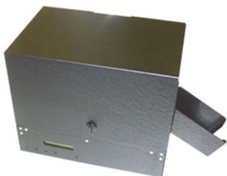
Boca-LM
