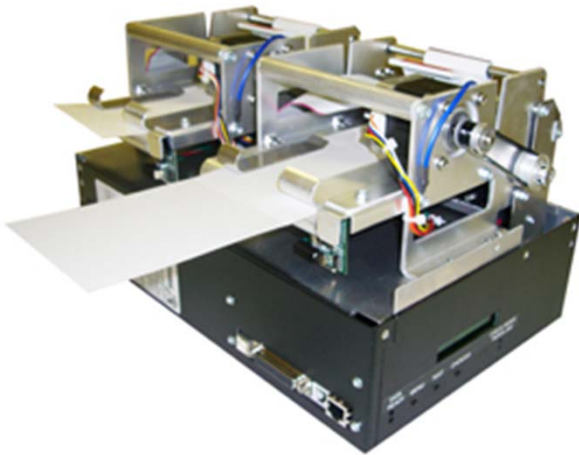
BOCA-L2K
